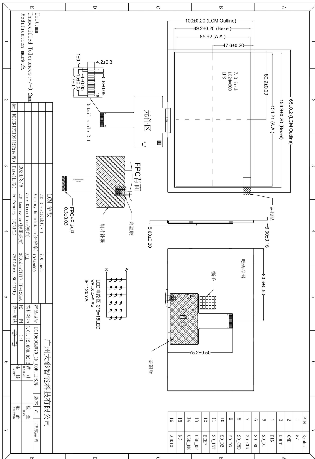
DC10600M070_1N_COF,IPS 屏尺寸图
