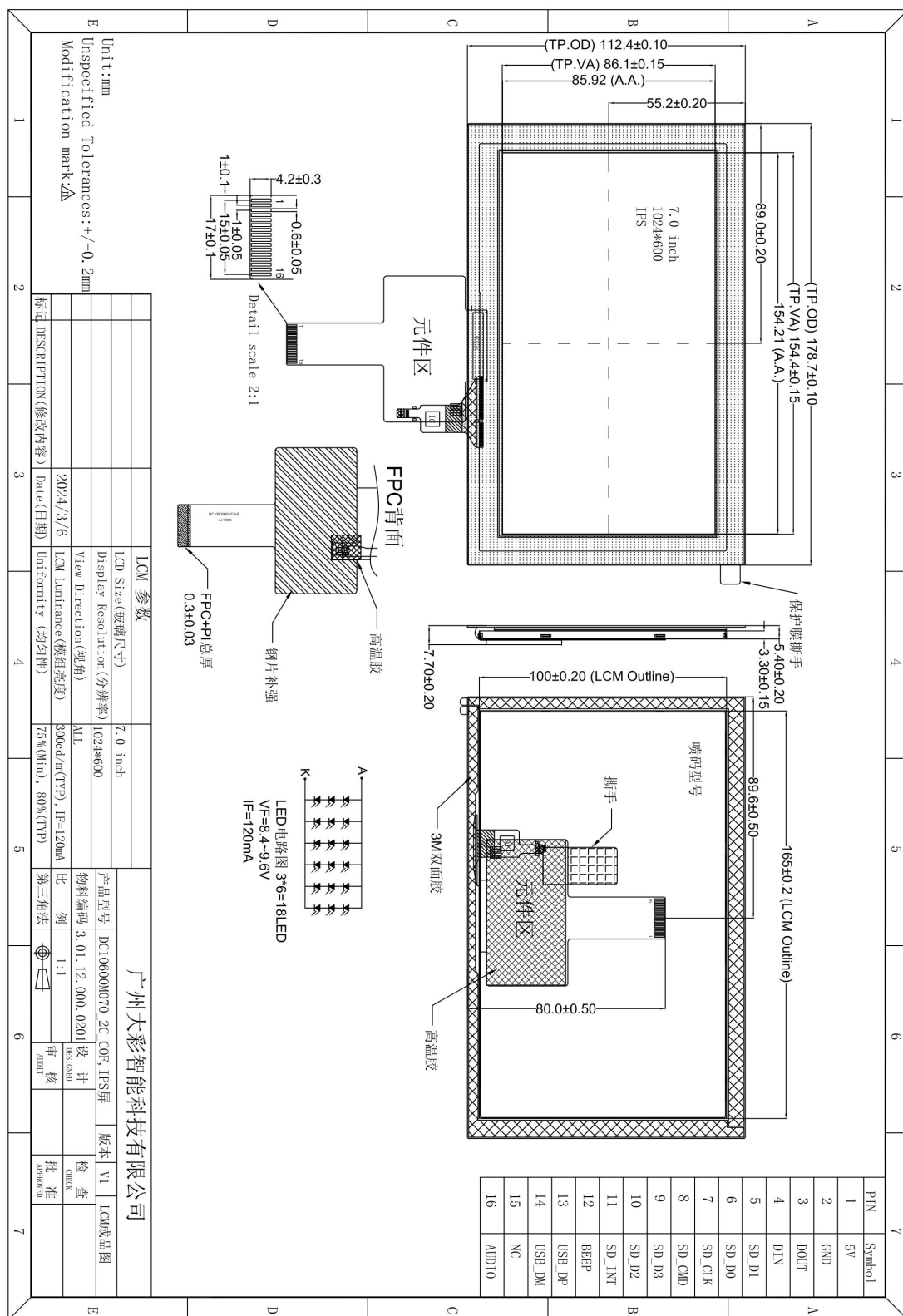
DC10600M070_2T_COF,IPS 屏尺寸图
