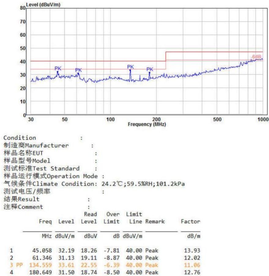
图 6-6 RE 测试垂直方向
