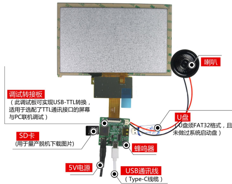
图 1-5 调试工具图
