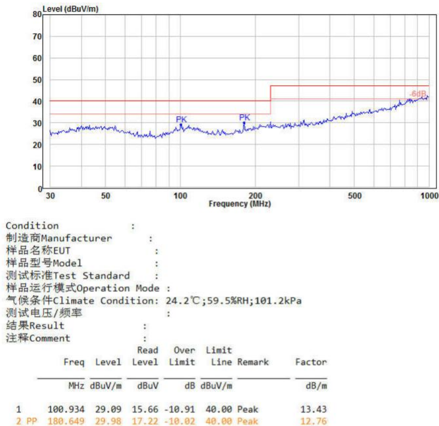
图 6-5 RE 测试水平方向
